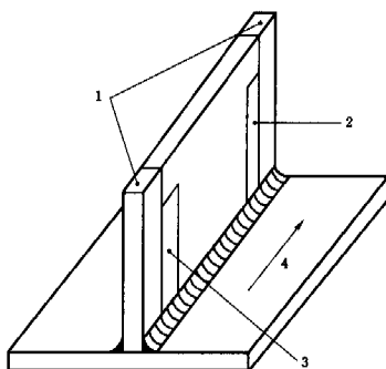
图 6 管子对接接头试样的位置
