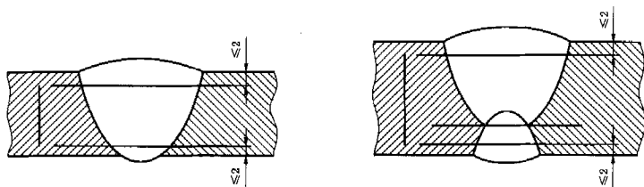
图 D.1 对接接头硬度测试点的选取
