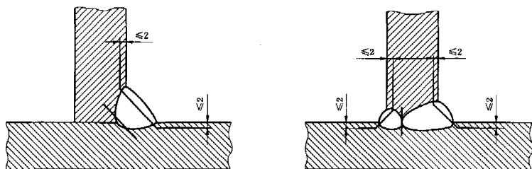
图 D.2 角焊接接头硬度测试点的选取
