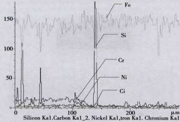
图 8 焊缝-20G 钢交界区线扫描各元素(Cr、Fe、Ni、Si、C)分布比较图
