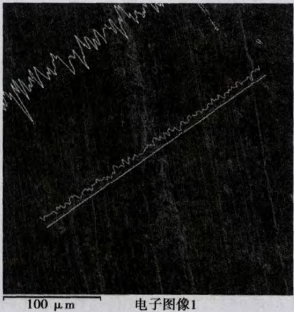
图 4 焊缝-316L 交界处线扫描元素示意图
