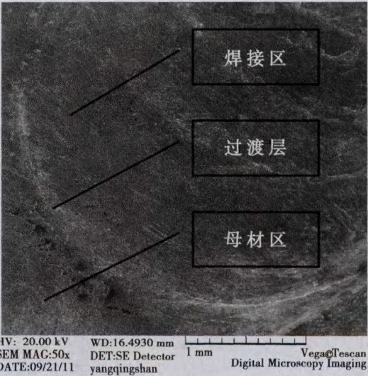
图 10 316L-20G 复合管焊缝的宏观形貌
