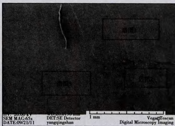
图 2 焊缝区-316L-20G 钢三者结合区域
