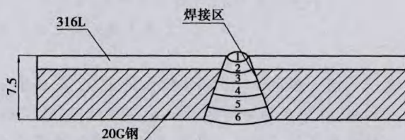
图 1 复合管焊缝区域示意图
