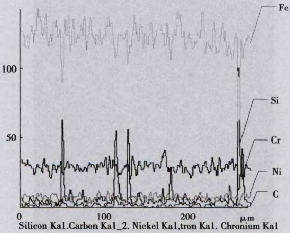
图 5 焊缝-316L 交界处线扫描元素(Cr、Fe、Ni、Si、C)分布对比图
