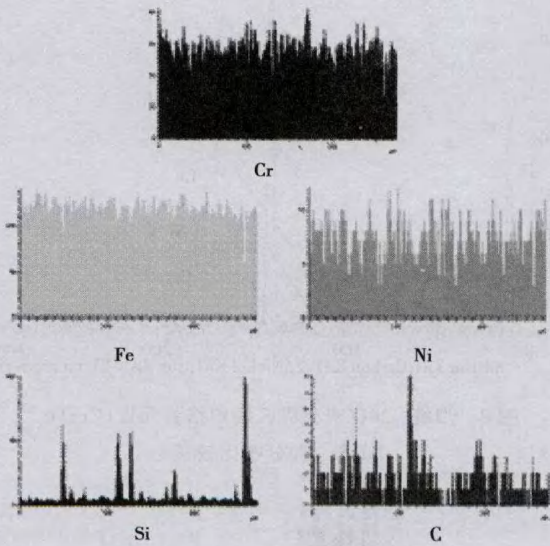
图 6 焊缝-316L 交界处线扫描各元素(Cr、Fe、Ni、Si、C)分布对比图
