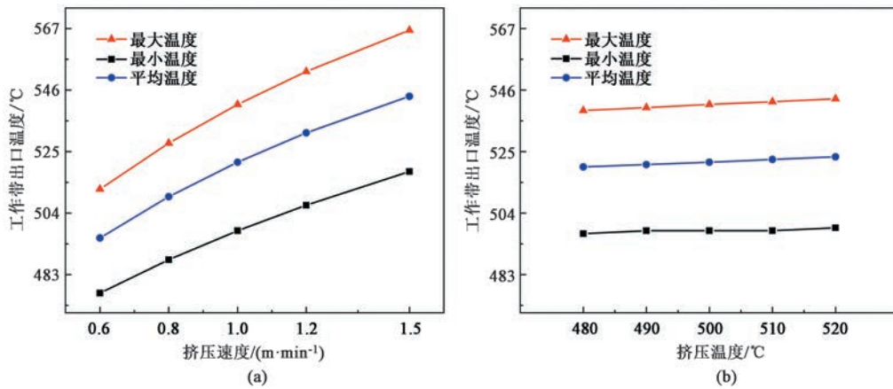
图 4 工艺参数对挤出型材温度分布的影响
