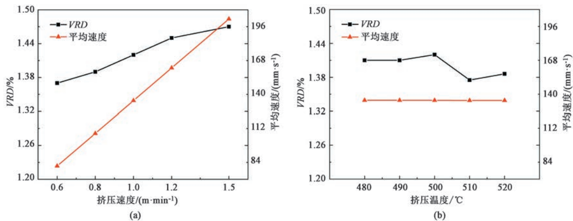
图3 工艺参数对工作带出口截面流速分布的影响
