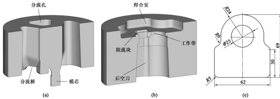
图 1 分流模剖面图和集流管截面尺寸 (a) 上模 (b) 下模 (c) 集流管横截面
