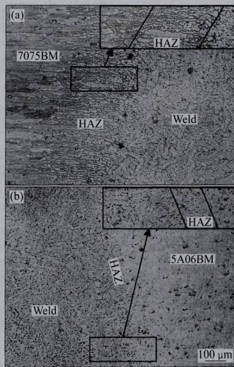
图3 采用 ER4043 焊丝获得的接头显微组织
