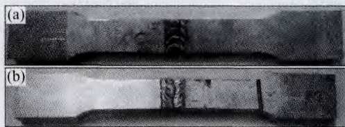
图6 接头断裂位置示意图
