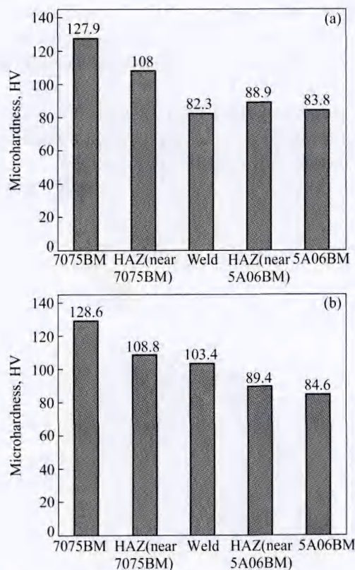
图8 采用 BJ380A 焊丝和 ER4043 焊丝获得的接头显微硬度分布
