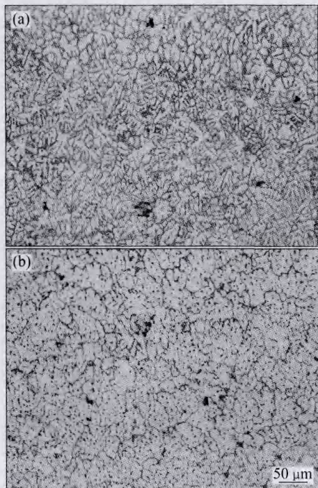
图4 采用 BJ380A 焊丝获得正面焊缝的显微组织
