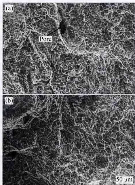
图7 采用 BJ380A 焊丝获得的接头断口 SEM 像
