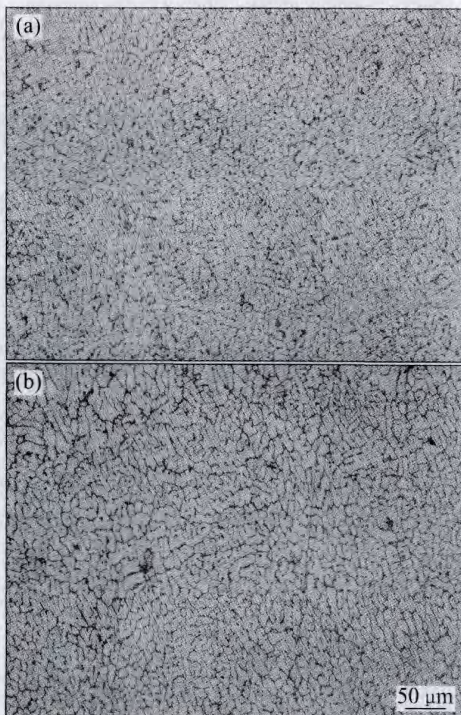
图5 采用 ER4043 焊丝获得正面焊缝的显微组织
