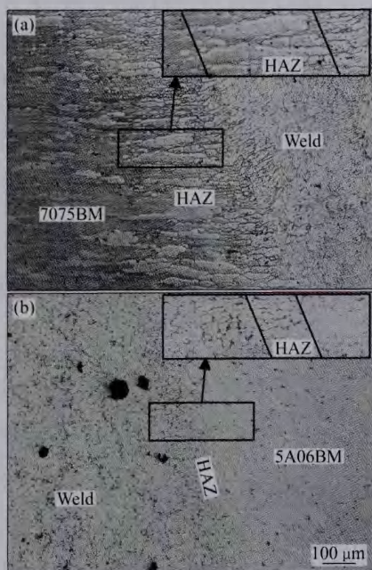
图2 采用 BJ380A 焊丝获得的接头显微组织
