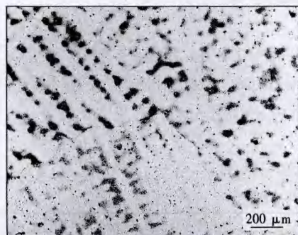
(c) 均匀化母材树枝晶与偏析区 (灰色)
