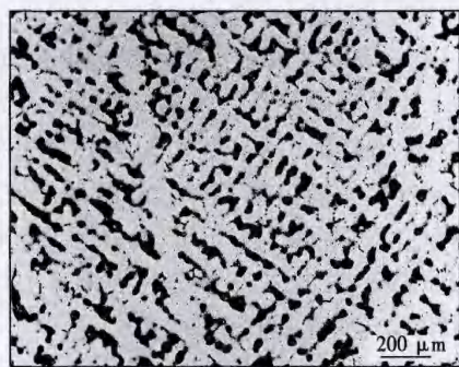
(b) 铸态母材树枝晶与偏析区 (黑色)
