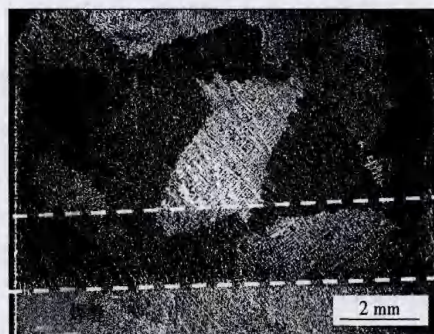
(b) 铸态母材焊接接头上表面金相 (2.4 kJ/cm)
