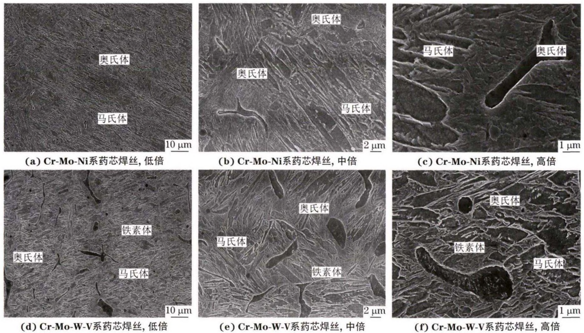
图2 不同药芯焊丝堆焊层的显微组织
