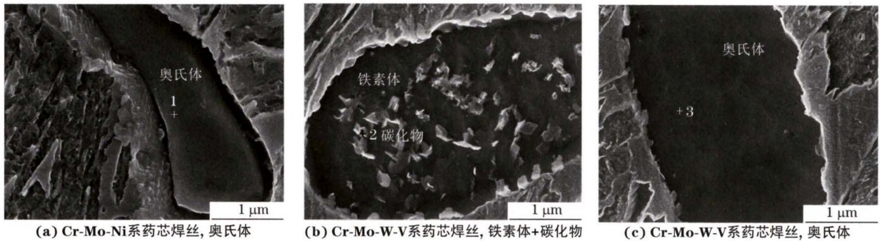
图3 不同药芯焊丝堆焊层的EDS分析位置
