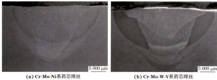
图1 不同药芯焊丝堆焊层的宏观形貌
