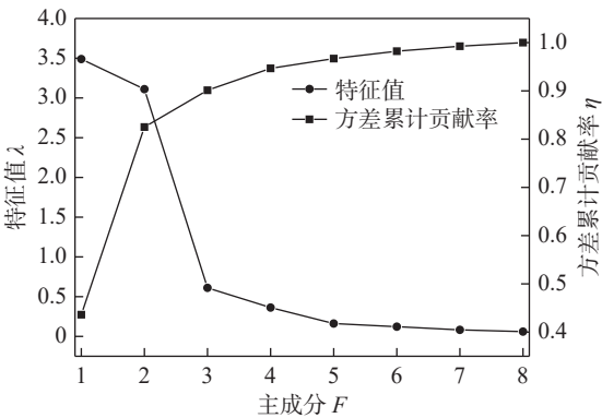
图 11 主成分分析结果 Fig. 11 Principal components analysis result
