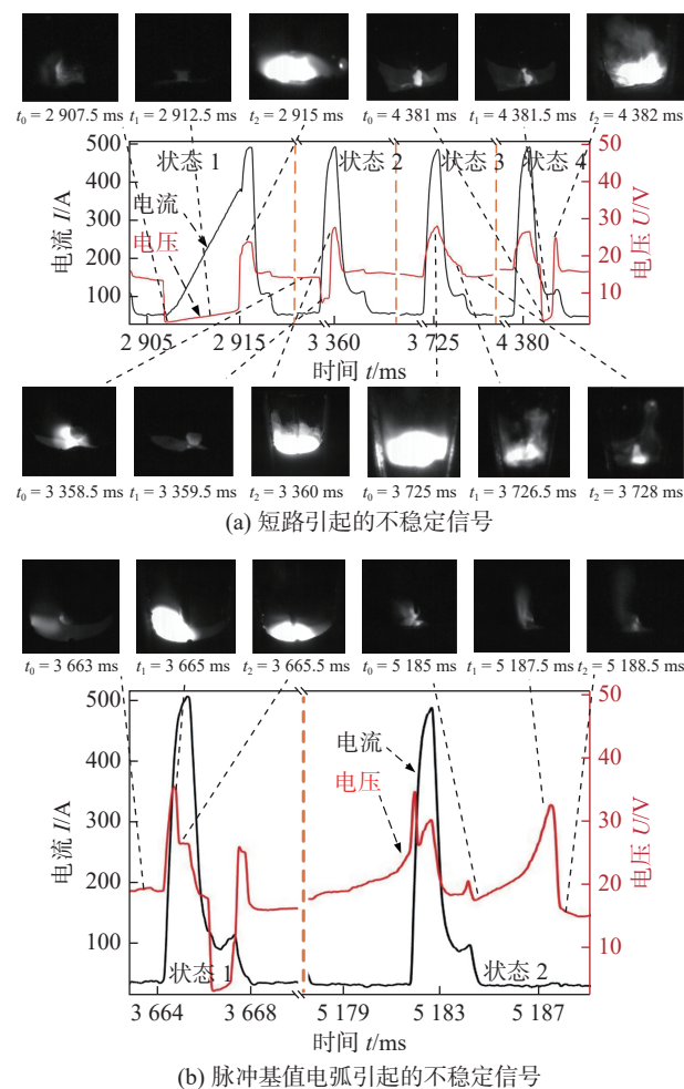
图 8 弧长调节阶段的电信号
