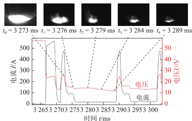
图 6 弧长较短时电信号
