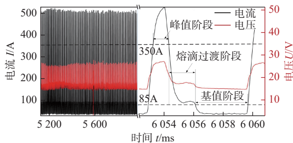
图 2 电信号脉冲波形 Fig. 2 Electric signal pulse waveform
