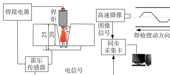
图 1 试验系统示意图 (mm) Fig. 1 Schematic diagram of experimental system
