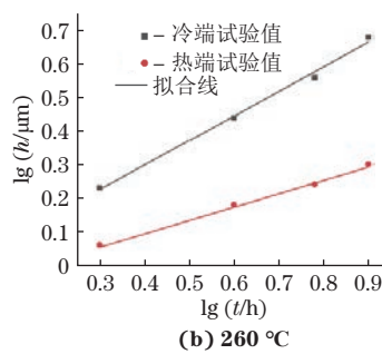
图8 不同回流温度下接头冷端和热端 \lg h - \lg t 拟合结果
