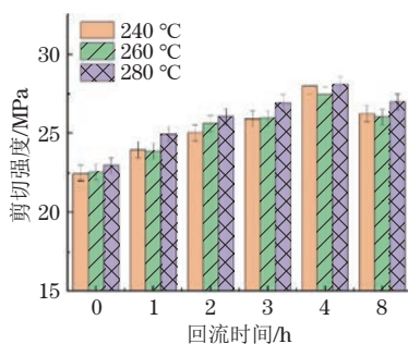
图 9 不同回流温度、不同回流时间下接头的剪切强度
