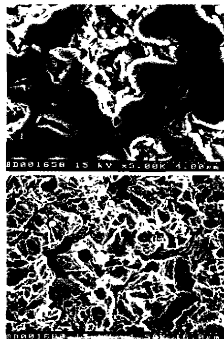
图1 CuNiSiB覆层材料的气蚀形貌
