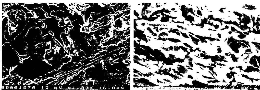
图 2 NiCrSiB 覆层材料的气蚀形貌
