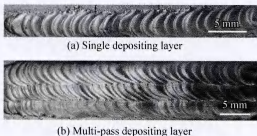
图1 镁合金再制造熔敷层宏观形貌
