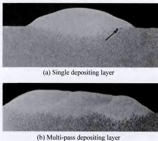
图2 镁合金再制造熔敷层截面形貌
