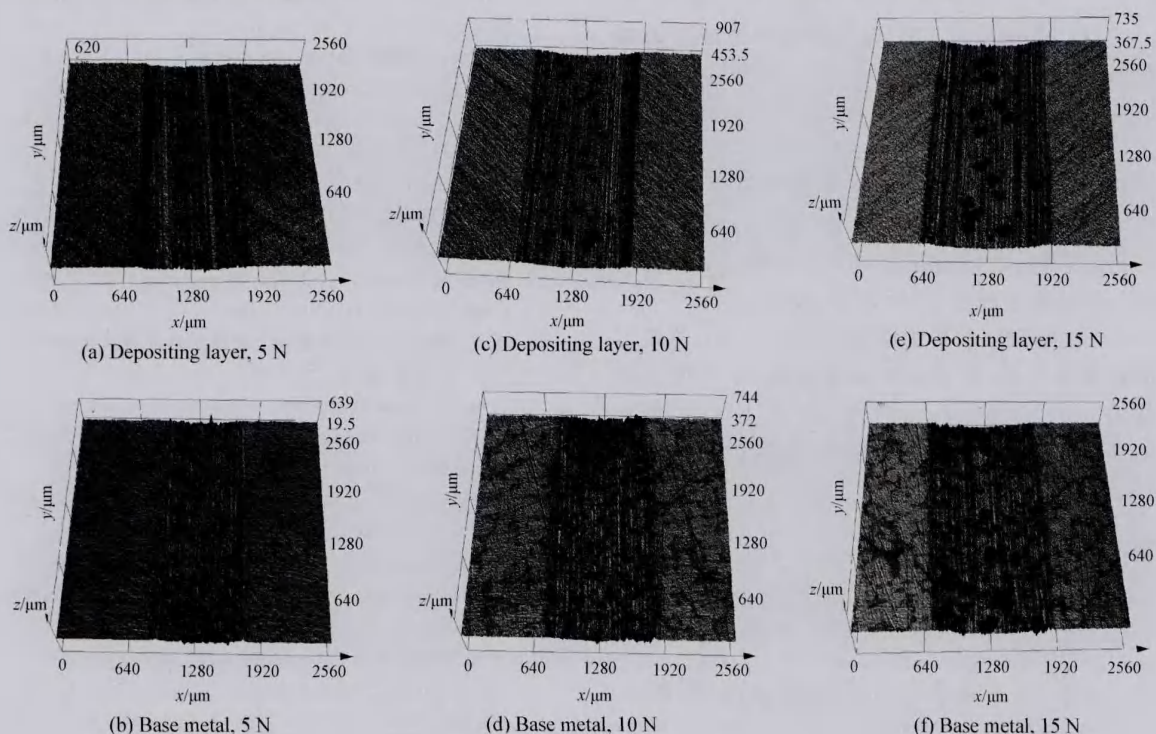
图 11 熔敷层与母材的三维磨痕形貌
