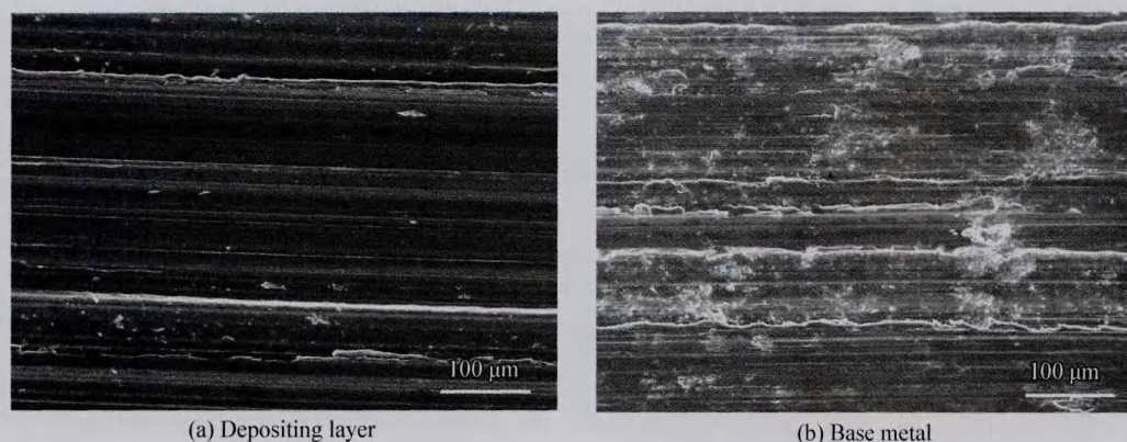
图 10 在 10 N 载荷下母材与熔敷层的磨痕形貌
