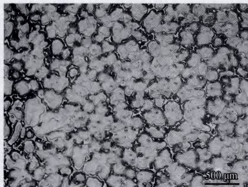
图3 ZM5 镁合金母材的微观组织
