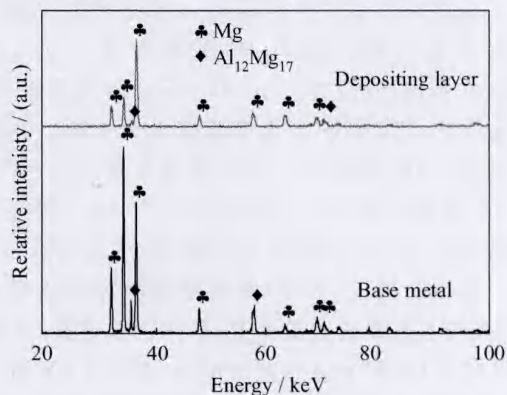
图5 母材与熔敷层XRD衍射图谱
