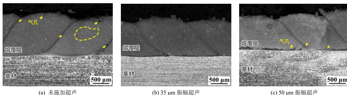
图2 不同条件下激光熔覆试样宏观形貌
