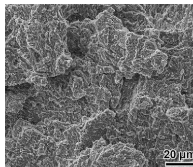
(b) 熔覆层
