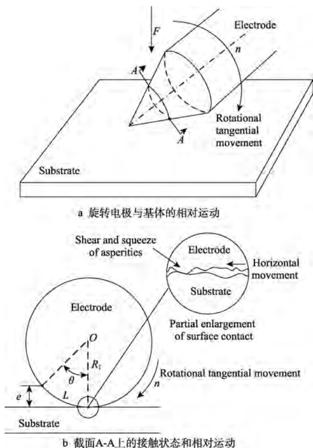
图 8 旋转电极与基体的接触状态和相对运动
