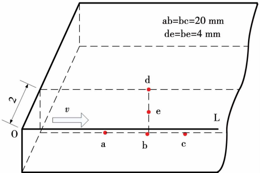
图 7 焊道上关键点示意图(mm)
