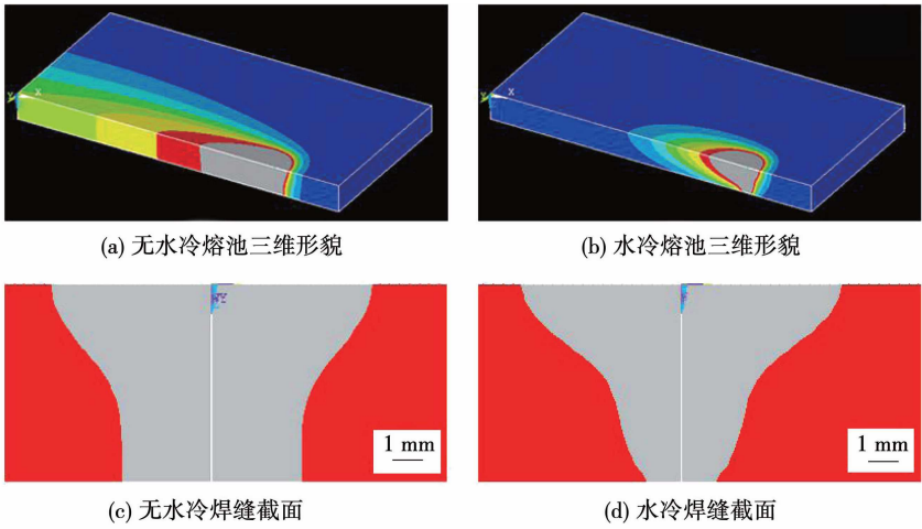
图 6 熔池三维图及焊缝截面示意图
