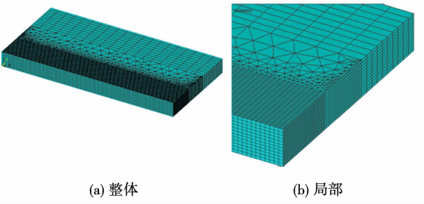
图 2 网格模型示意图 Fig. 2 Diagram of mesh model
