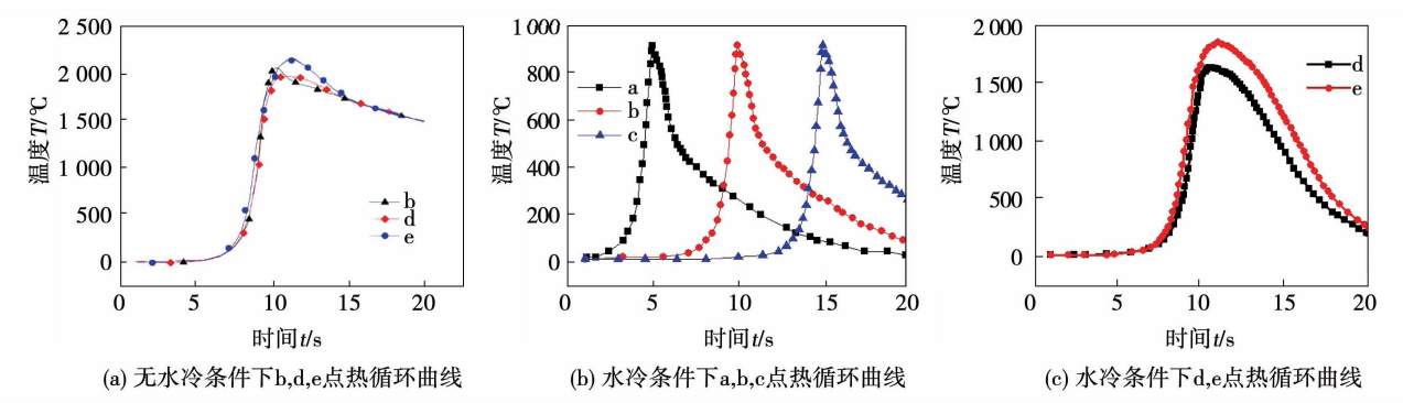
图 8 热循环曲线示意图 Fig. 8 Diagram of thermal cycle cruve
