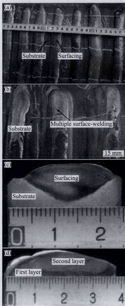
图 3 复合涂层的宏观形貌
