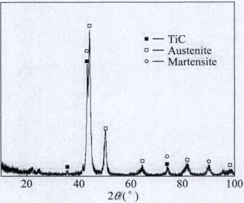
图 4 复合涂层的 XRD 谱 Fig.4 XRD pattern of composite coating
