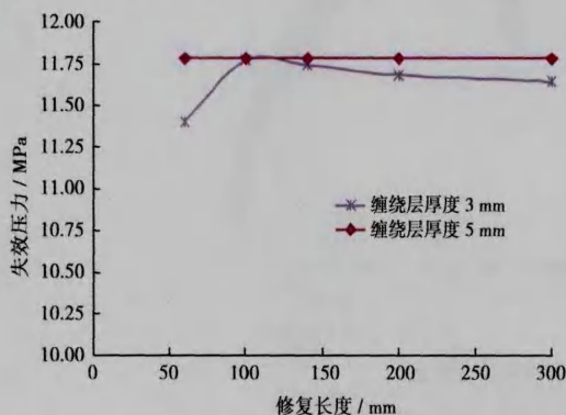
图 10 失效压力与缠绕层长度关系
