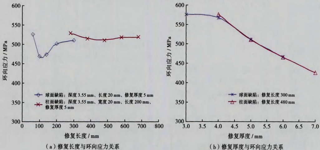
图 9 X60 管道不同修复长度和厚度对应的缠绕层最大环向应力
