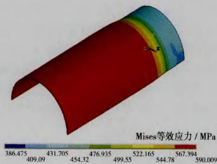
图5 极限状态下算例1管道 Mises 等效应力云图
