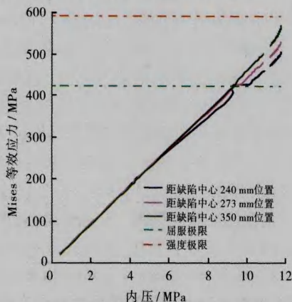
图6 缠绕层附近管体应力与内压的关系
