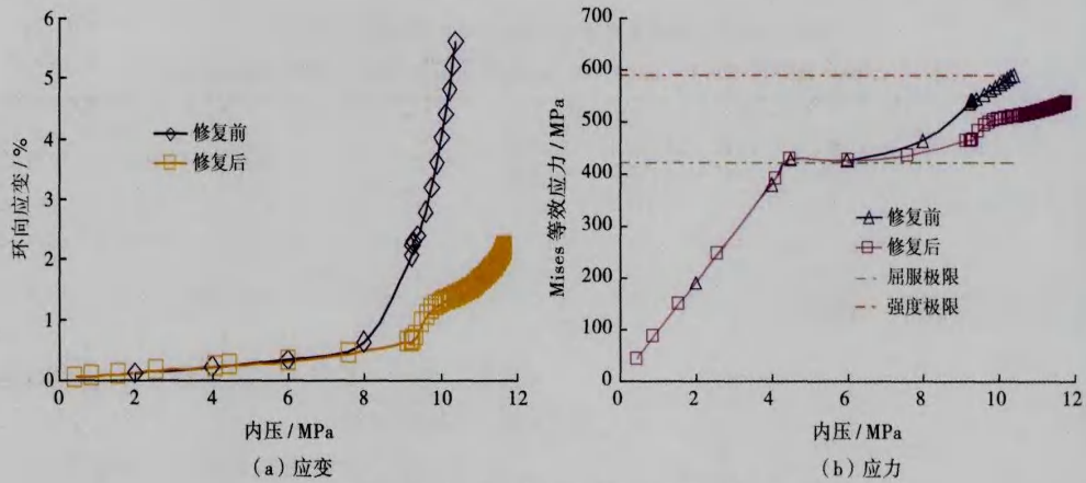
图4 算例1管道修复前后的应力与应变
