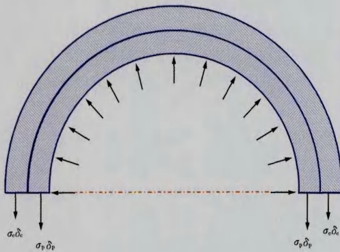
图1 缠绕补强管段的受力状态
