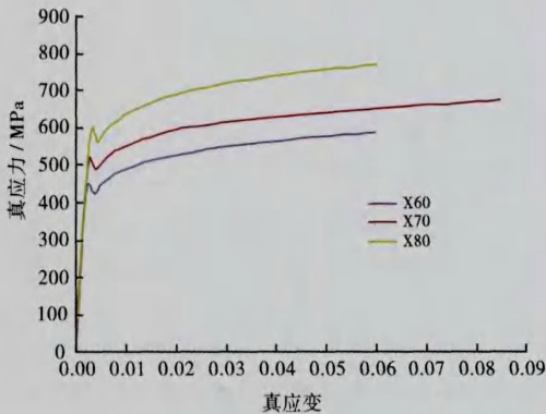
图 3 X60、X70 和 X80 管材应力-应变曲线
