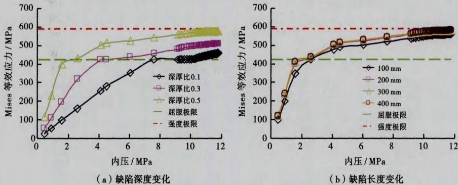
图 8 算例 1 管道缺陷中心处应力与内压的关系
