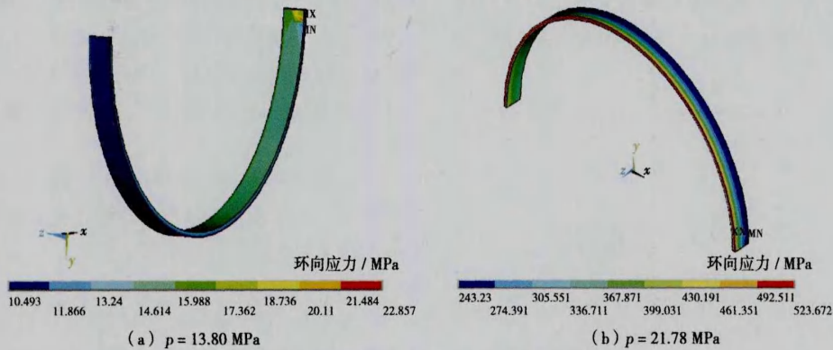
图 7 算例 3 管道缠绕层中的环向应力云图
