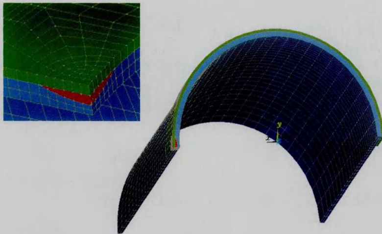
图 2 含缺陷修复管道有限元模型
