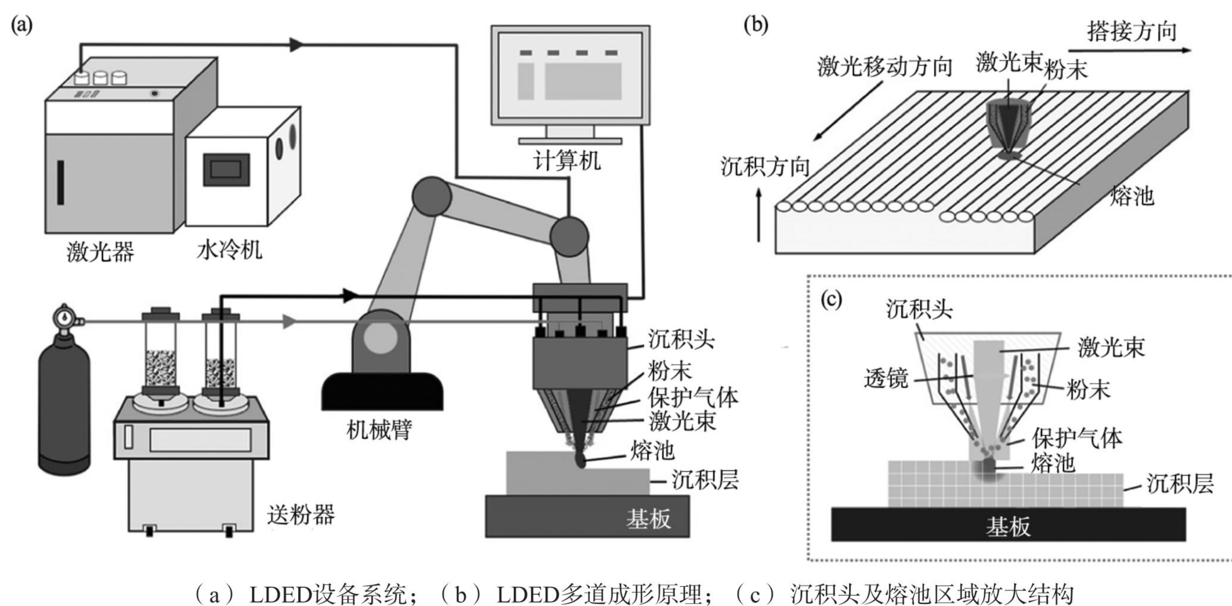
图2 LDED设备及工作示意图
