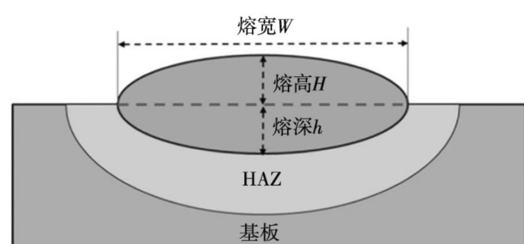
图3 熔池几何参数示意图
