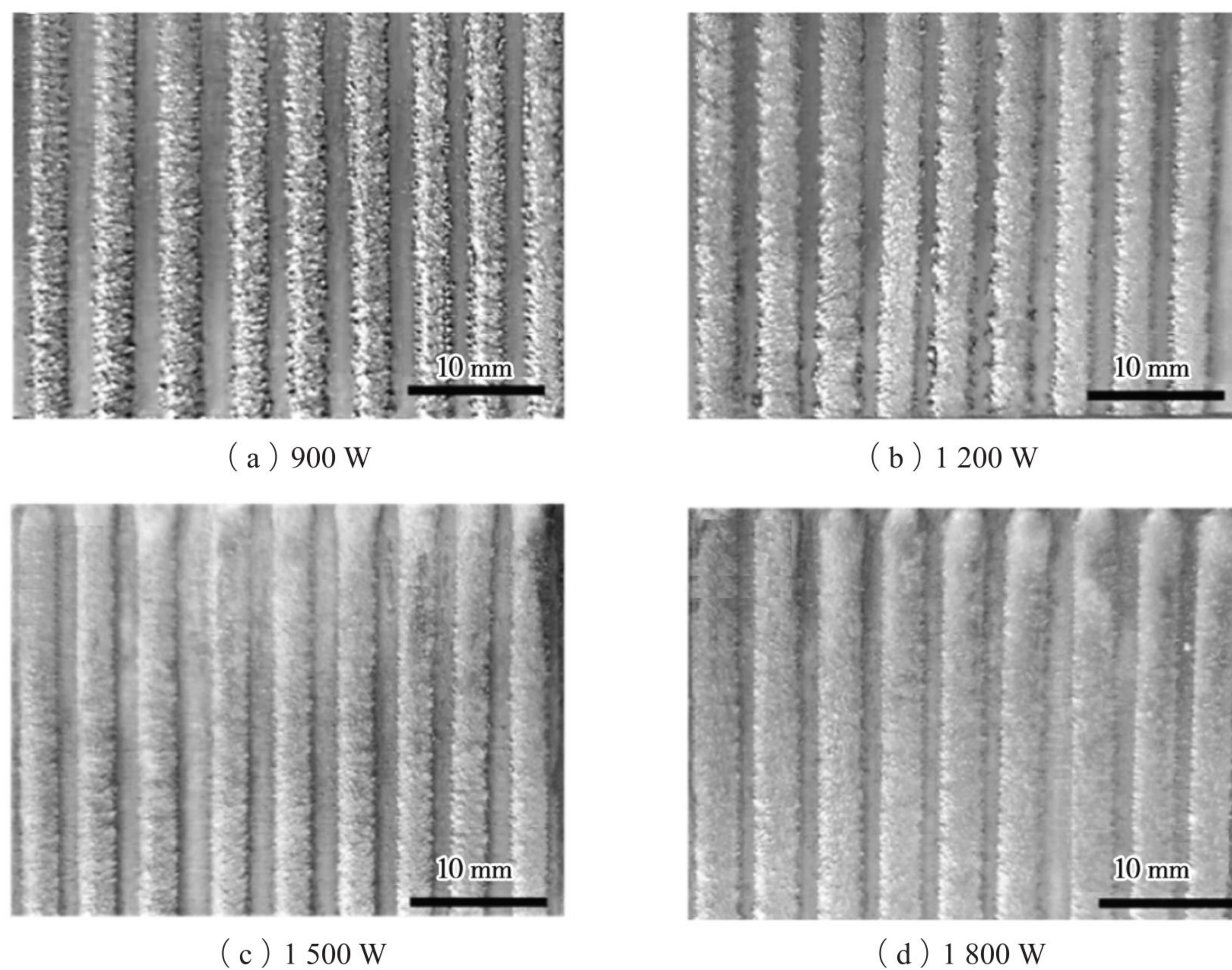
图4 不同参数下单道表面形貌
