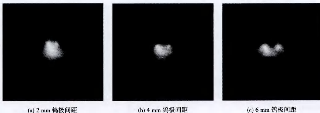
图 10 不同钨极间距时的电弧形貌
