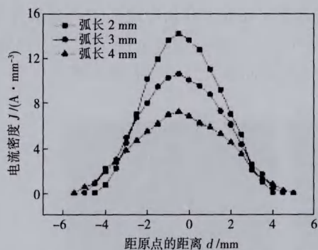
图6 弧长对阳极电流密度分布的影响
