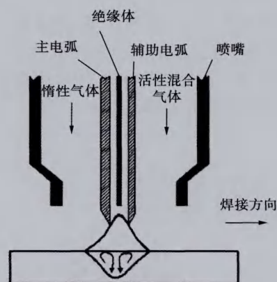
图 1 耦合电弧 AA-TIG 焊接示意图
