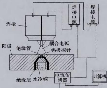
图2 阳极电流密度测量系统
