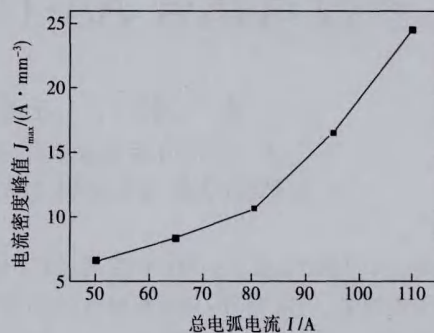
图4 总电弧电流对阳极电流密度峰值的影响
