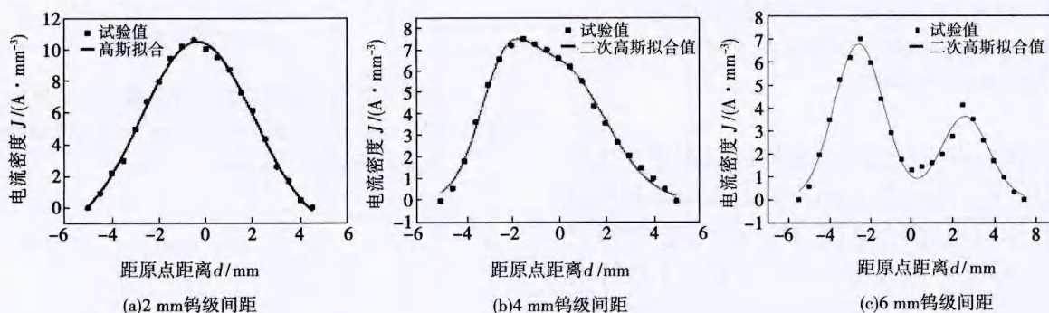
图 11 不同钨极间距时的阳极电流密度分布高斯拟合
