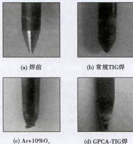
图 4 钨极氧化程度比较
