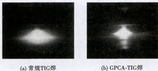
图 1 焊接电弧形态 Fig. 1 Arc shapes
