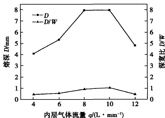
图9 内层气体流量对焊缝熔深及深宽比的影响
