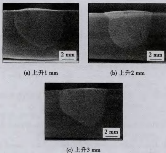
图5 外喷嘴不同的上升高度时焊缝截面形貌
