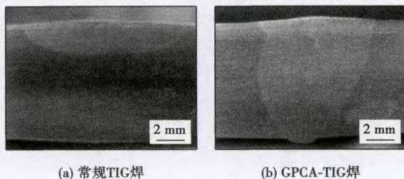
图 3 焊缝横截面形貌
