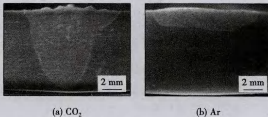
图7 外层气体种类对焊缝熔深熔宽的影响
