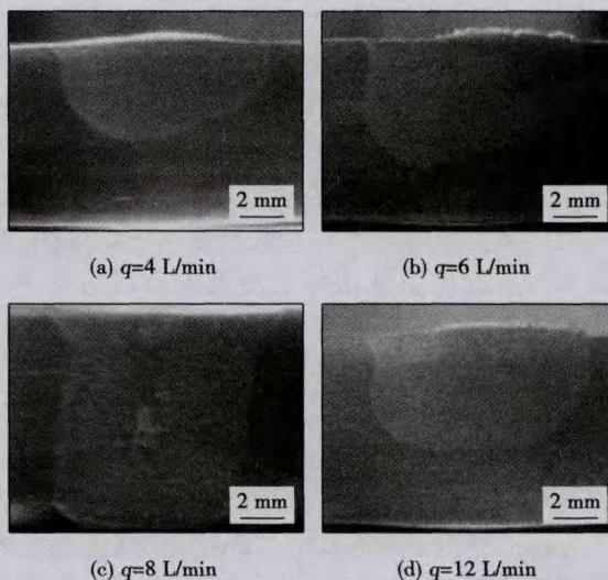
图8 不同内层气体流量时焊缝截面形貌
