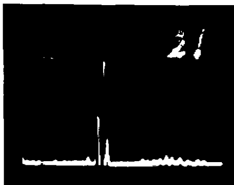
图 6 铜体裂纹波形
