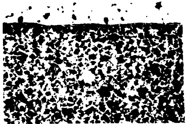
图 4 结合面钢基体组织 117×
