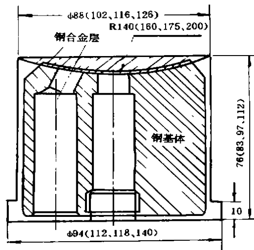
图 1 双金属转子零件、毛坯图
