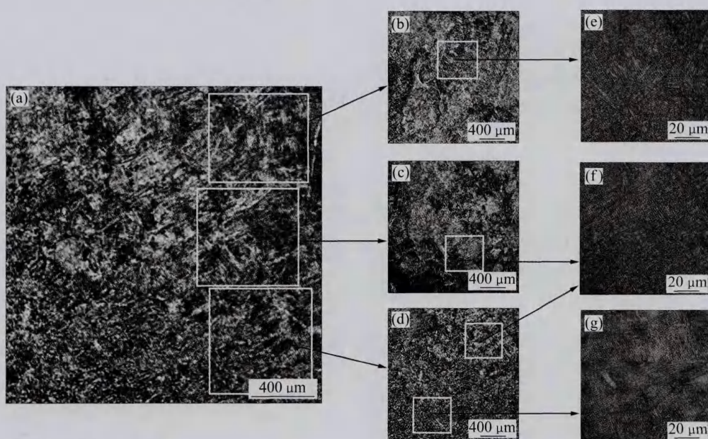
图7 无磁场作用时的焊缝组织
