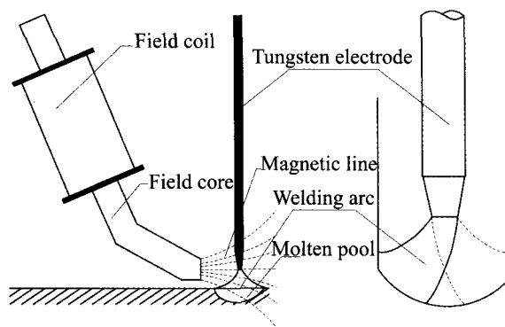
图1 窄间隙磁控电弧焊接方法示意图
