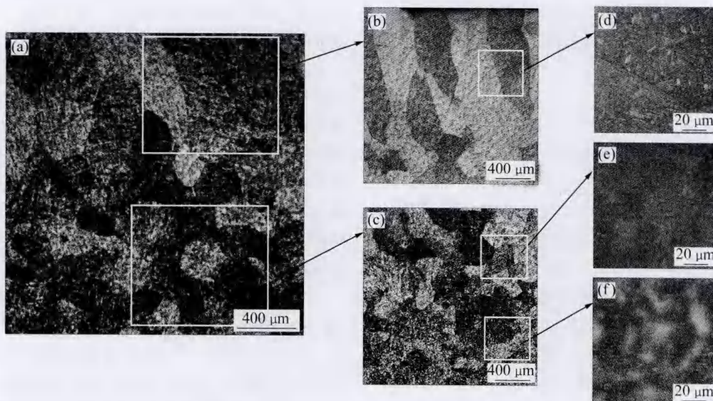
图6 8 mT、10 Hz 磁场作用时的焊缝组织
