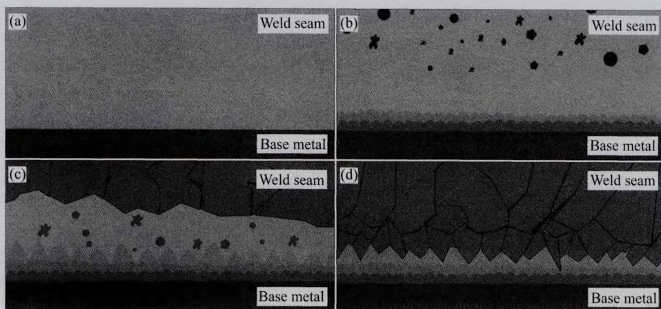
图8 磁场作用下钛合金焊缝金属一次结晶过程示意图
