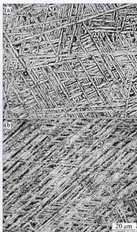
图 4 焊缝区的显微组织
