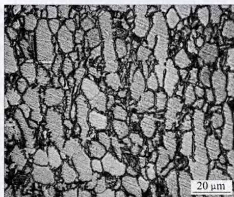
图 3 Ti-6Al-4V 钛合金的显微组织形貌
