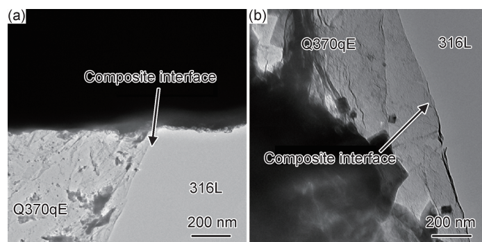
图4 不同终轧温度时不锈钢复合板界面区 TEM 图
