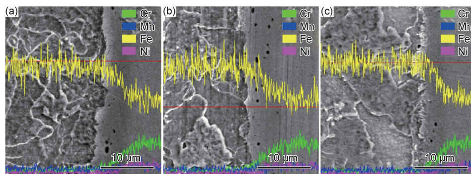
图3 不同终轧温度时不锈钢复合板界面区EDS线扫描结果
