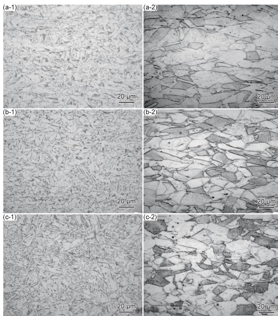
图5 不同终轧温度时不锈钢复合板碳钢基体(1)和不锈钢基体(2)显微组织
