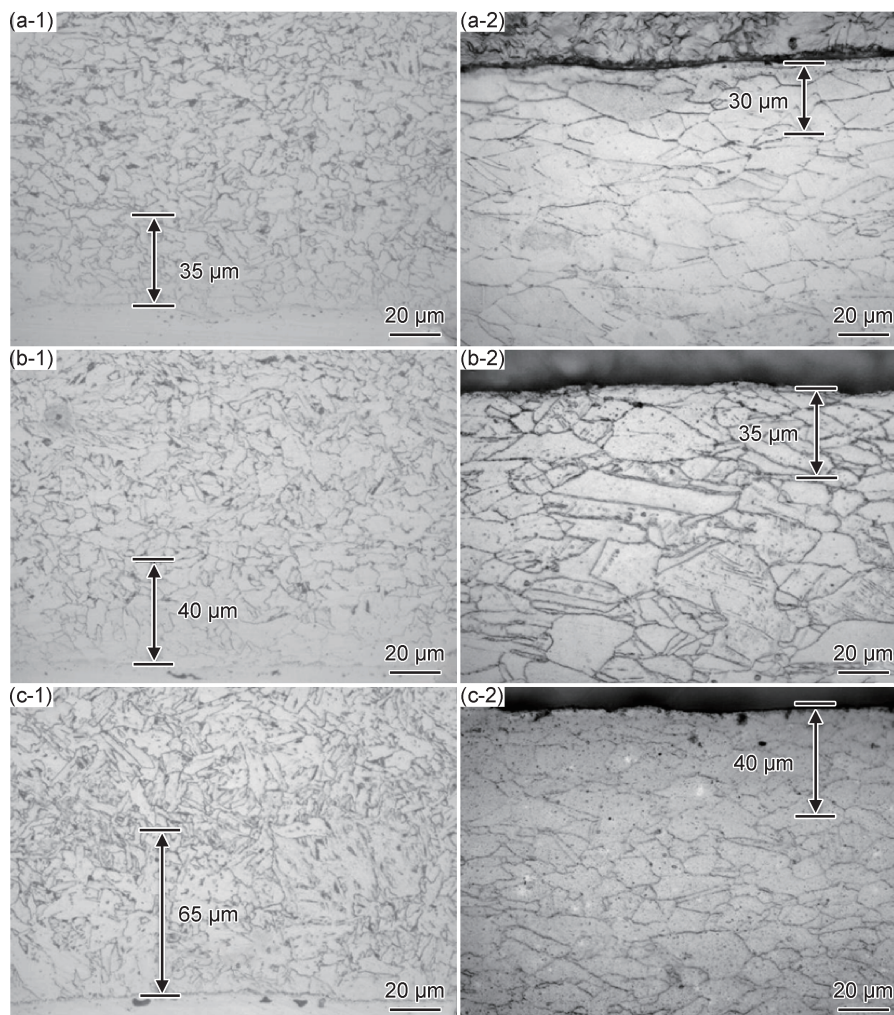
图2 不同终轧温度时不锈钢复合板界面区碳钢侧(1)和不锈钢侧(2)显微组织
