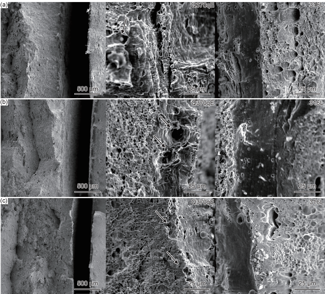
图8 不同终轧温度时不锈钢复合板拉伸断口形貌 (a)800℃;(b)840℃;(c)880℃
