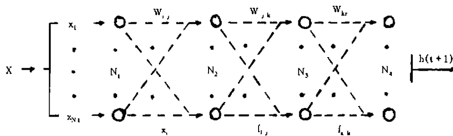
图 3 熔宽过程神经网络模型
