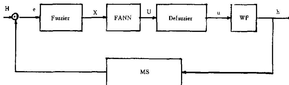
图 1 脉冲 TIG 焊熔宽模糊神经网络控制系统
