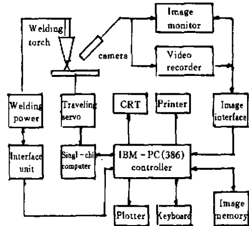
图 5 试验系统硬件框图
