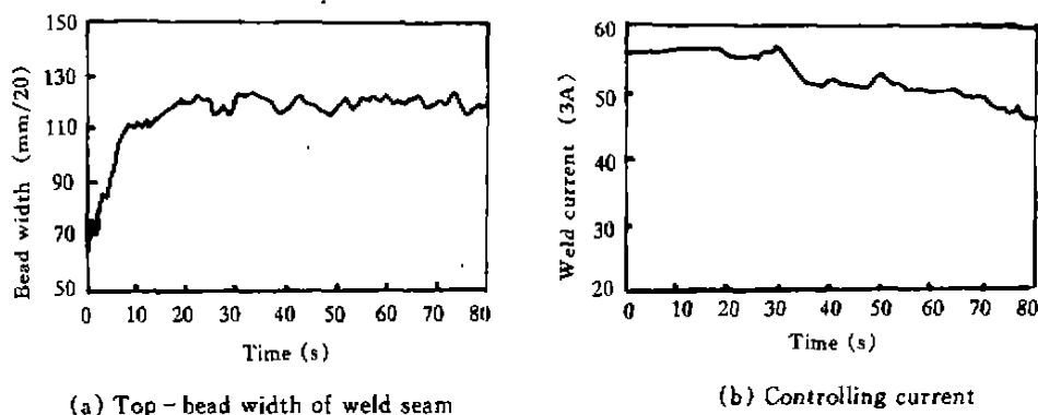
图 8 模糊神经网络控制结果
