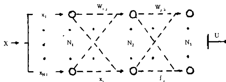
图 2 模糊神经网络控制模型
