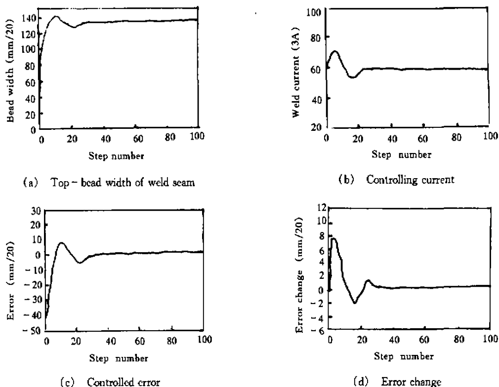
图 4 控制方案的仿真结果
