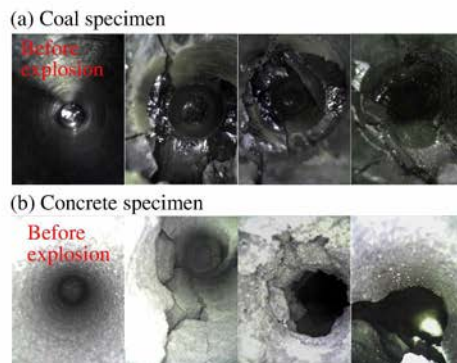
图7 爆孔内裂隙分布
