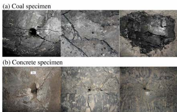
图6 裂隙形貌分布
