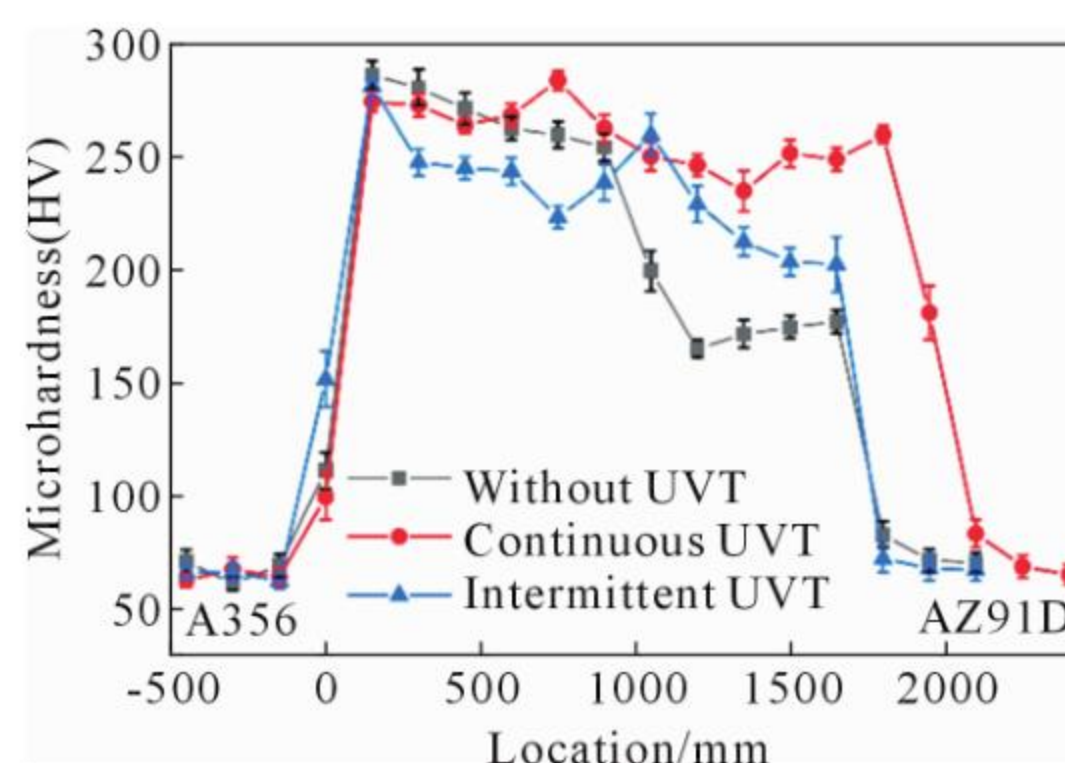
图6 Al/Mg 双金属界面显微硬度分布
