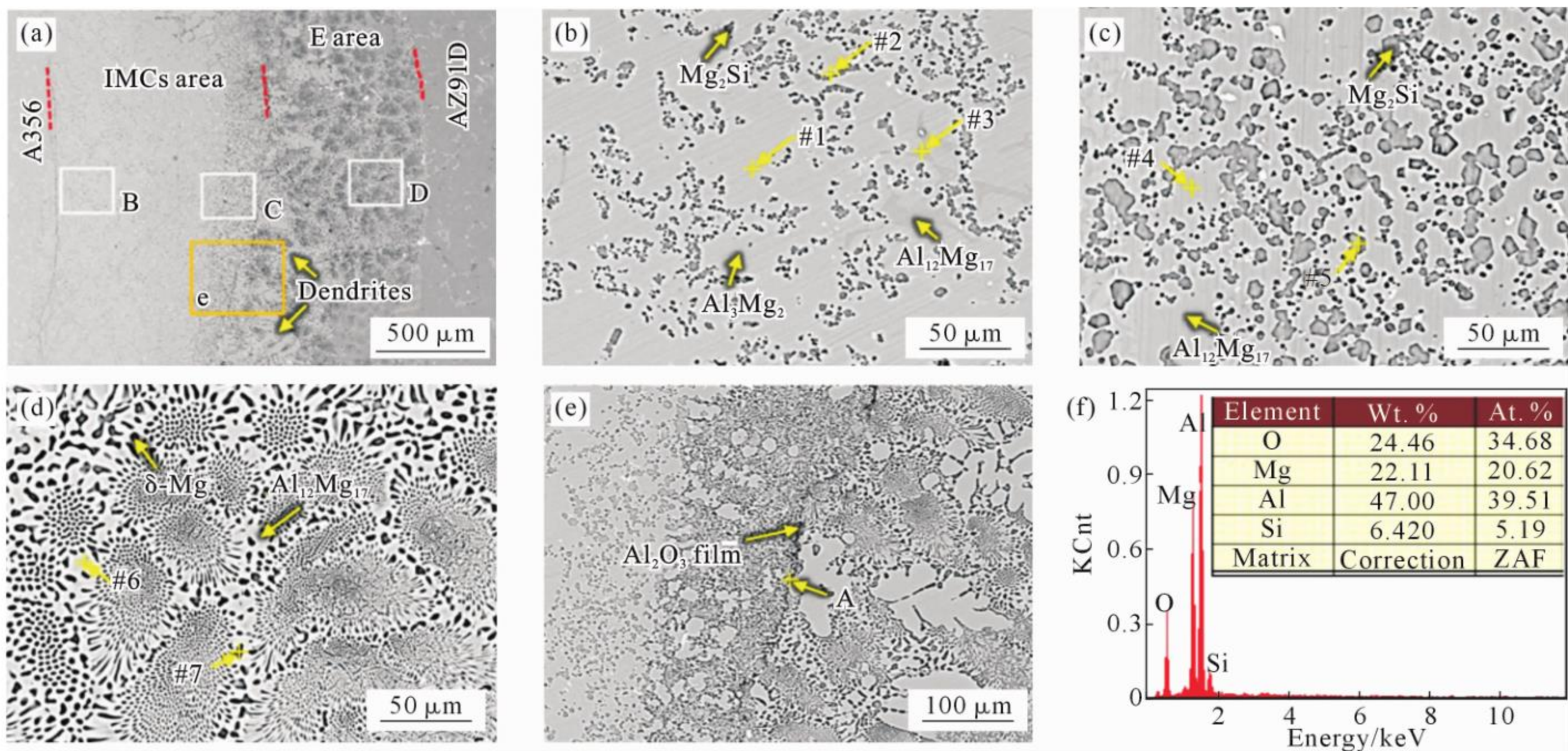
图 3 不施加超声振动 Al/Mg 双金属界面形貌与不同区域微观组织:(a) 整体形貌;(b) (a)中 B 区域高倍图;(c) (a)中 C 区域高倍图;(d) (a)中 D 区域高倍图;(e) 金属间化合物区和共晶组织区边界氧化膜;(f) (e)中 A 点 EDS 结果
