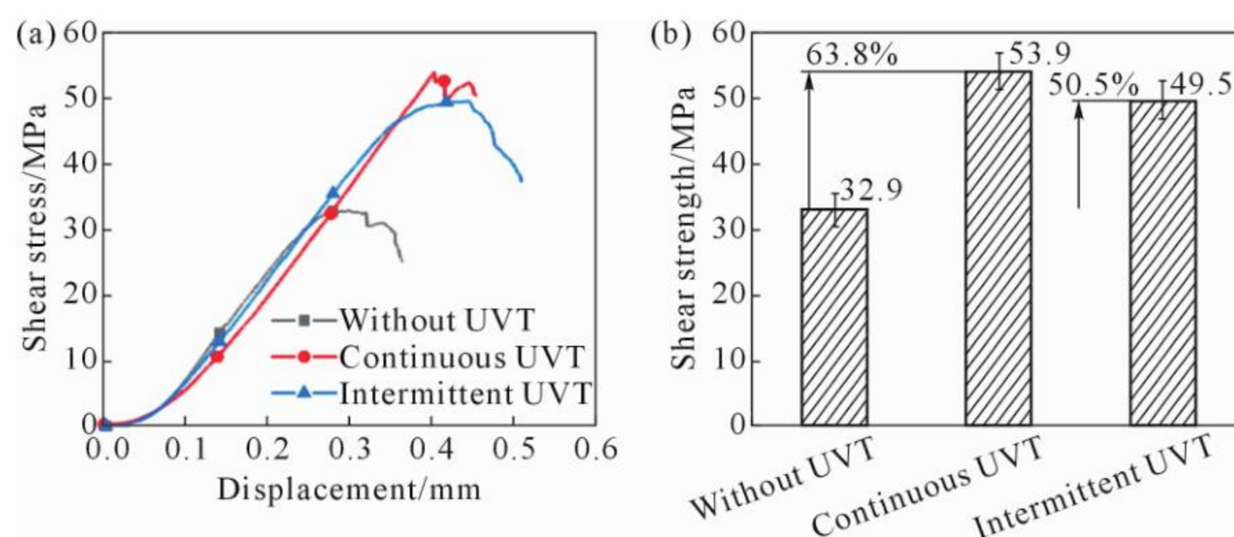
图 7 Al/Mg 双金属界面的剪切性能: (a)剪切应力-位移曲线; (b)剪切强度
