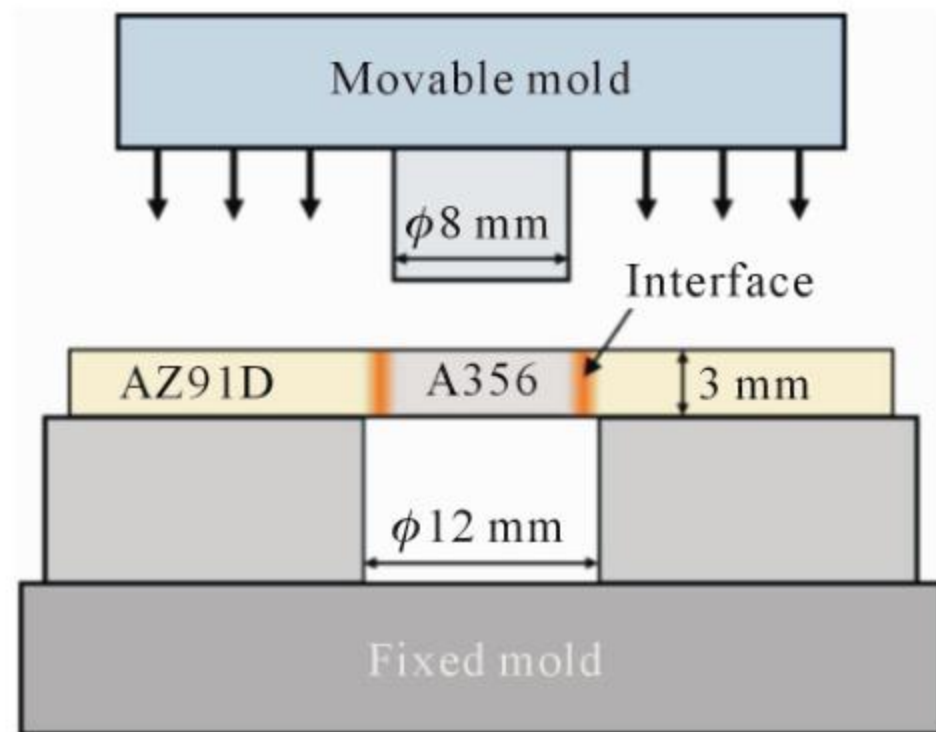
图 2 Al/Mg 双金属材料剪切测试示意图
