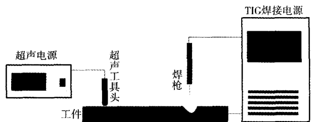
图 1 试验装置示意图 Fig. 1 Schematic of experimental device
