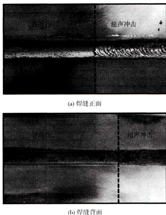
图 4 间断超声对焊缝成形影响
